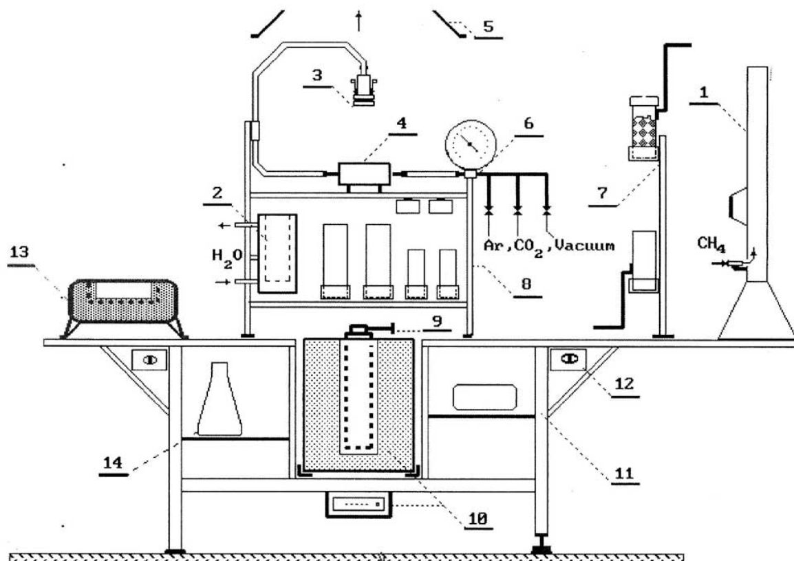
Scheme of benzene line (High temperature). Схема бензоловой линии (Высокотемпературная часть).
